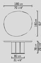
OLLE Dining table 180x160 cm PBC 03.13--
